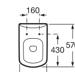
Miska WC podwieszana*
